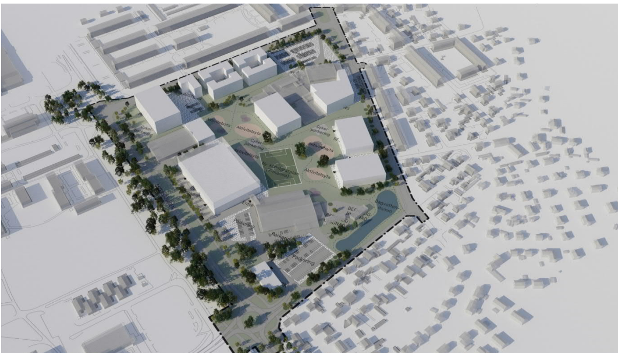
Höstdagjämning kl. 15
