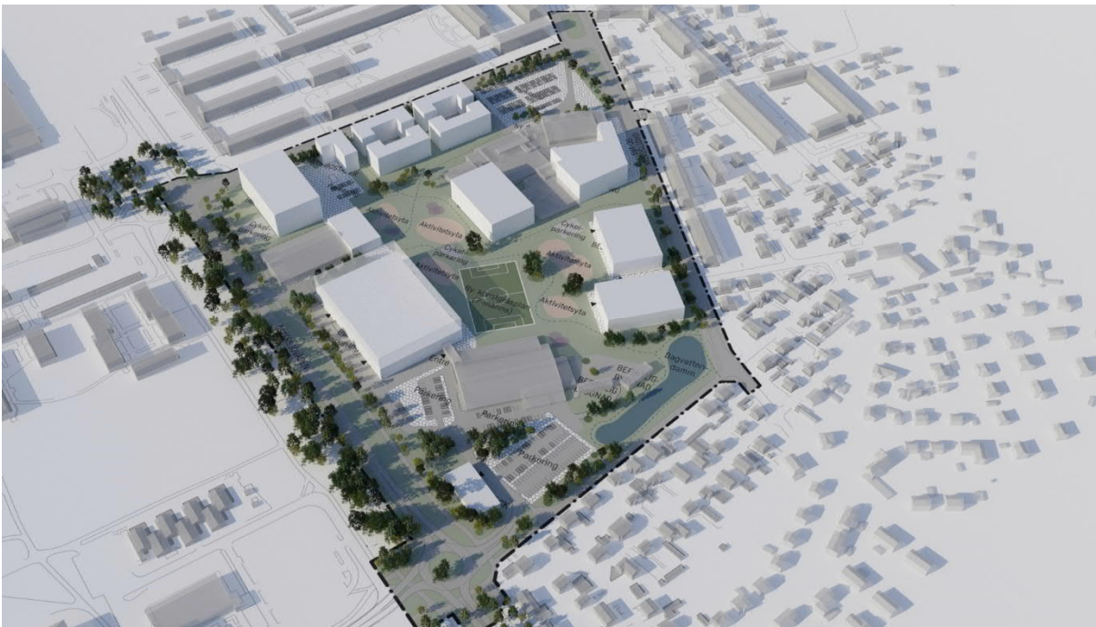
Vårdagjämning kl. 15
