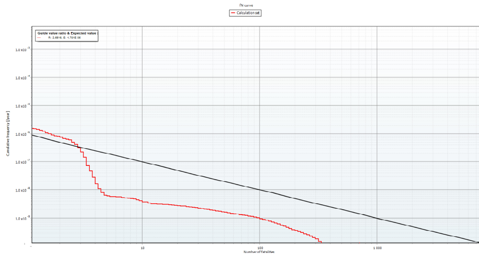
Figur 5. FN-kurva som visar samhällsrisken i närheten av anläggningen. Svart rät linje visar nedre gränsen i ALARP-området.
