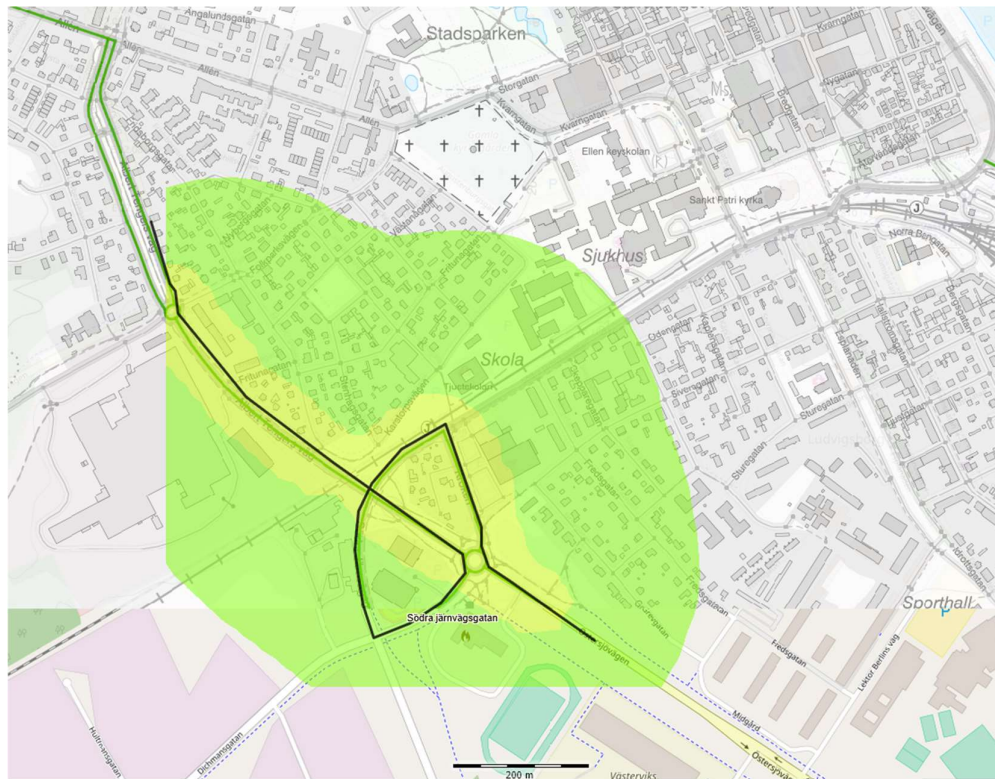
Figur 6. Samhällsrisken i form av riskkonturer markerade på en karta där gul markering illustrerar risknivån inom den lägre delen av ALARP-gränsen och grön markering understiger ALARP-gränsen och därmed acceptabla risker.
