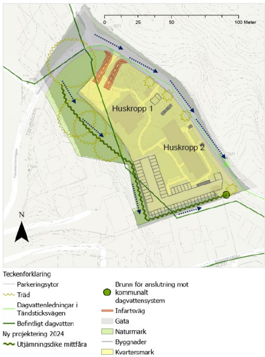
Figur 6: Principförslag till dagvatten- och skyfallshantering
