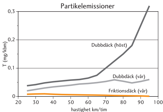
Hastighetens och årstidens betydelse för partikelemissioner.
